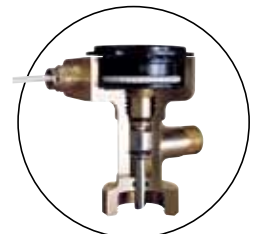
Patentierter, servounterstützter Zündkopf
